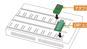
DIP ユニット装着例
